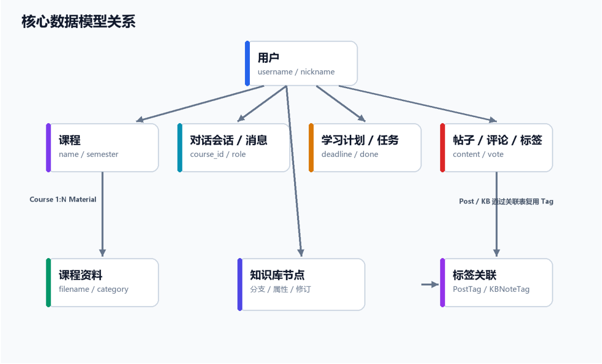
图 3-3 核心数据模型关系图
